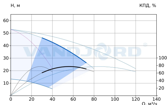
75111276 Hydro-ME 3 CRVE 32-3-2 G2-B-D-150-16-A
