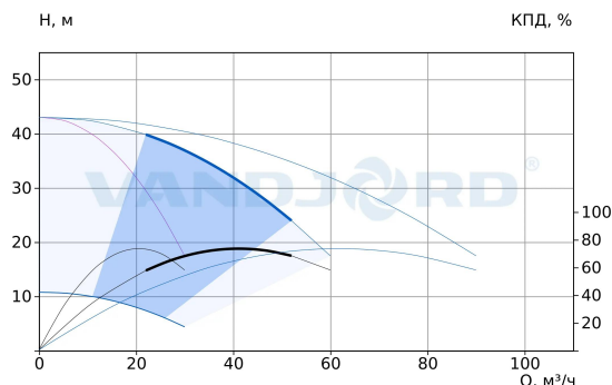
75111118 Hydro-ME 3 CRVE 20-3 G2-B-D-100-16-A
