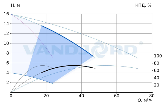
75111267 Hydro-ME 3 CRVE 15-1 G2-B-D-100-16-A
