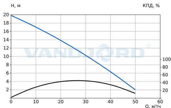
76122002 PROLIFT PD.22.3.150
