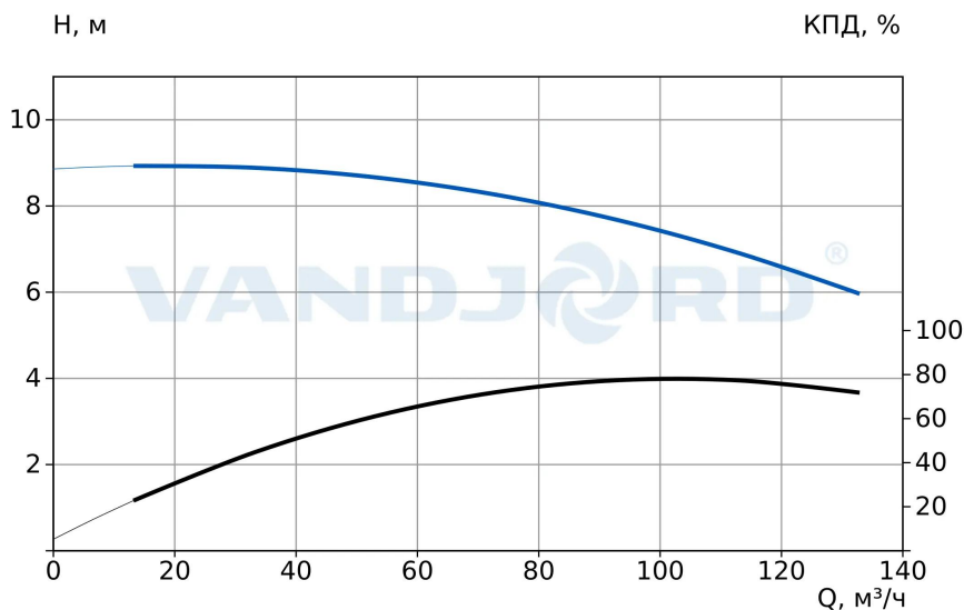
73118143 TPV 125-70-3/4 Q-A-BT-E
