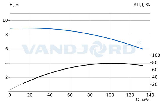
73118143 TPV 125-70-3/4 Q-A-BT-E
