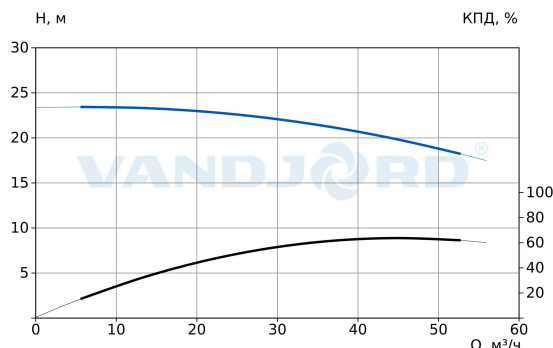
73115136 TPV 65-200-4/4 Q-A-BT-E
