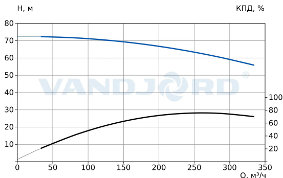
73118135 TPV 125-600-75/2 Q-A-BT-E
