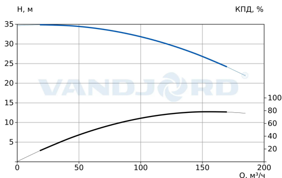
73117136 TPV 100-270-15/2 Q-A-BT-E
